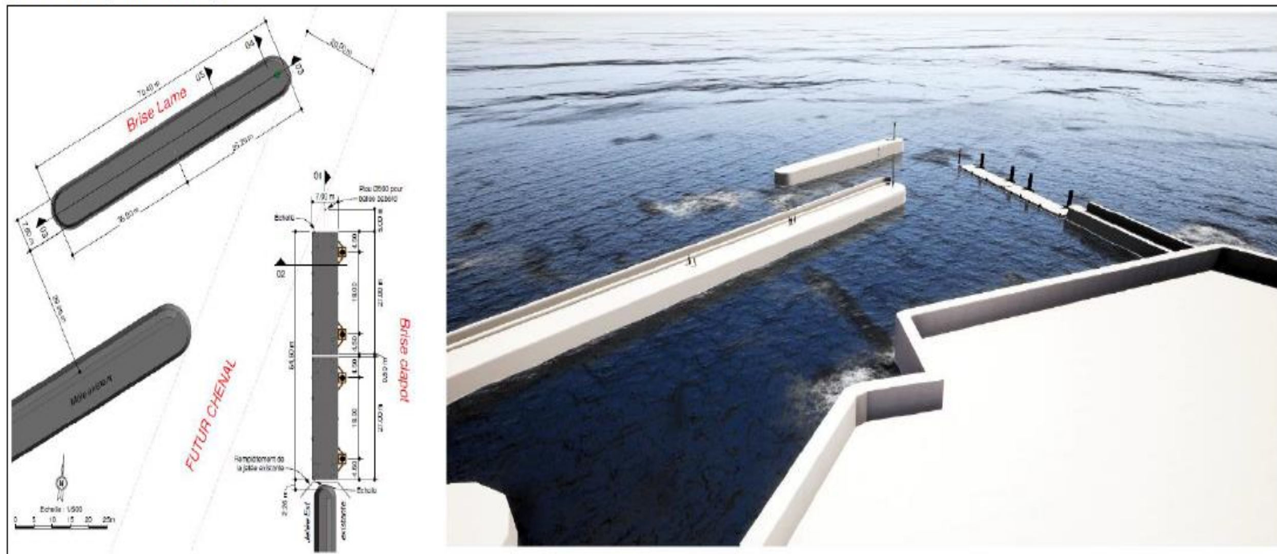
Figure 12 : Plan d'implantation des ouvrages.
